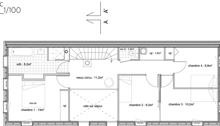
Plan 1er Etage Echelle _1/100
