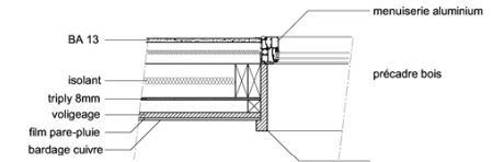
Détail 2 Echelle _1/20
