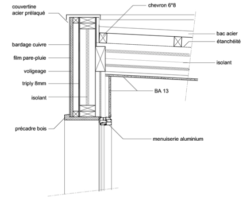
Détail 1 Echelle _1/20
