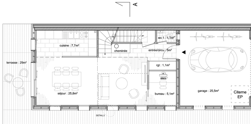
Plan Rdc Echelle _1/100
